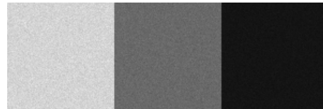
\lambda = 1000 (dose)
