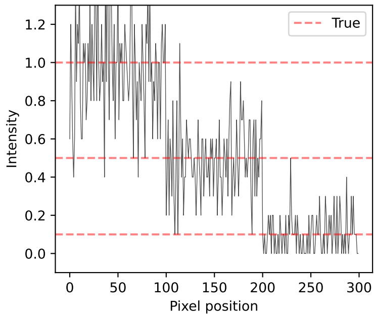
SNR: 3.2×
