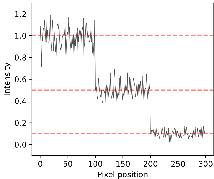
SNR: 10.0×
